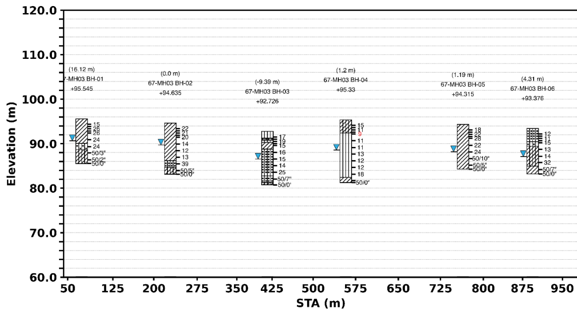
รูปที่ 32 ตัวอย่างภาพตัดขวางชั้นดินที่ได้จากการใช้คำสั่ง Rendering Soil Profile
