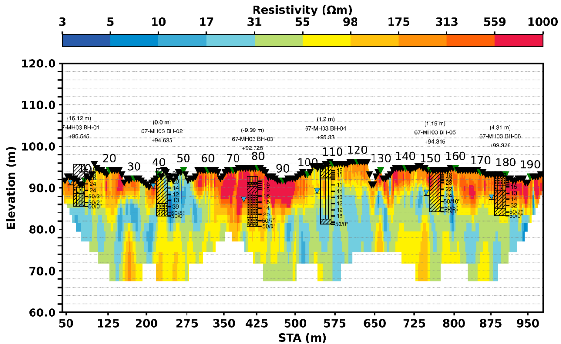
รูปที่ 31 ตัวอย่างแบบจำลองค่าสภาพต้านทานไฟฟ้าพร้อมข้อมูลหลุมเจาะ
